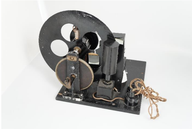
Fernsehempfänger nach Nipkow, Modell
